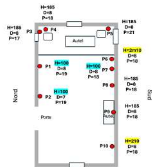
Plan rectangulaire a vaisseau unique.
